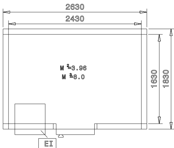
Boční
