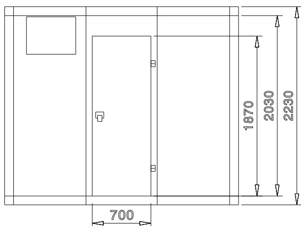
Boční
